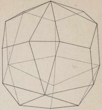
15. Penta-Tetraeder.
