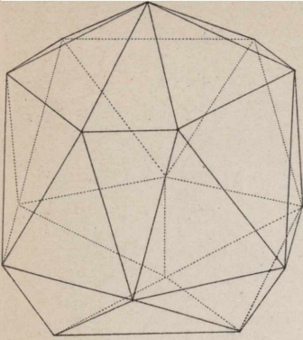
14. Tetra-Tetraeder.
