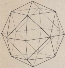
11. Pyramiden-Hexa-Tetraeder.
