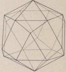
10. Hexa-Tetraeder.
