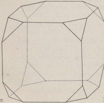
Tetra-Octaeder.
