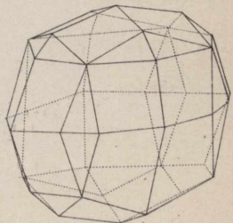
15. Amphieder.
