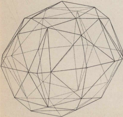
17. Octocontaeder.
