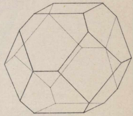
10. Hexa-Tetraeder.
