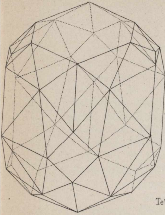
1. Heptacontaeder.
