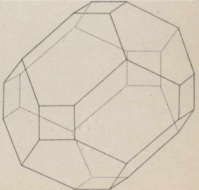
18. Octo-Tetraeder.
