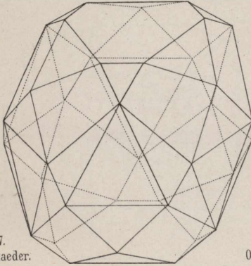
16. Pentacontaeder.
