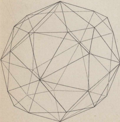
Penta-Octaeder.
