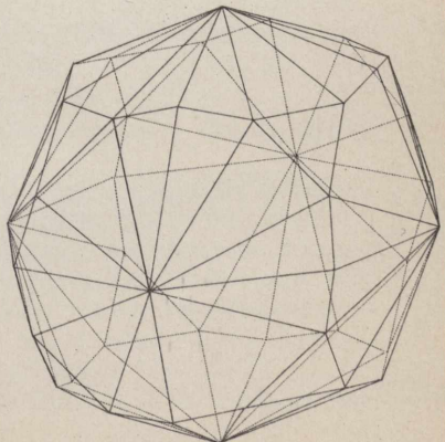
Hepta-Octaeder.
