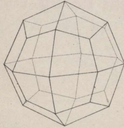
12. Würfel-Hexa-Tetraeder.
