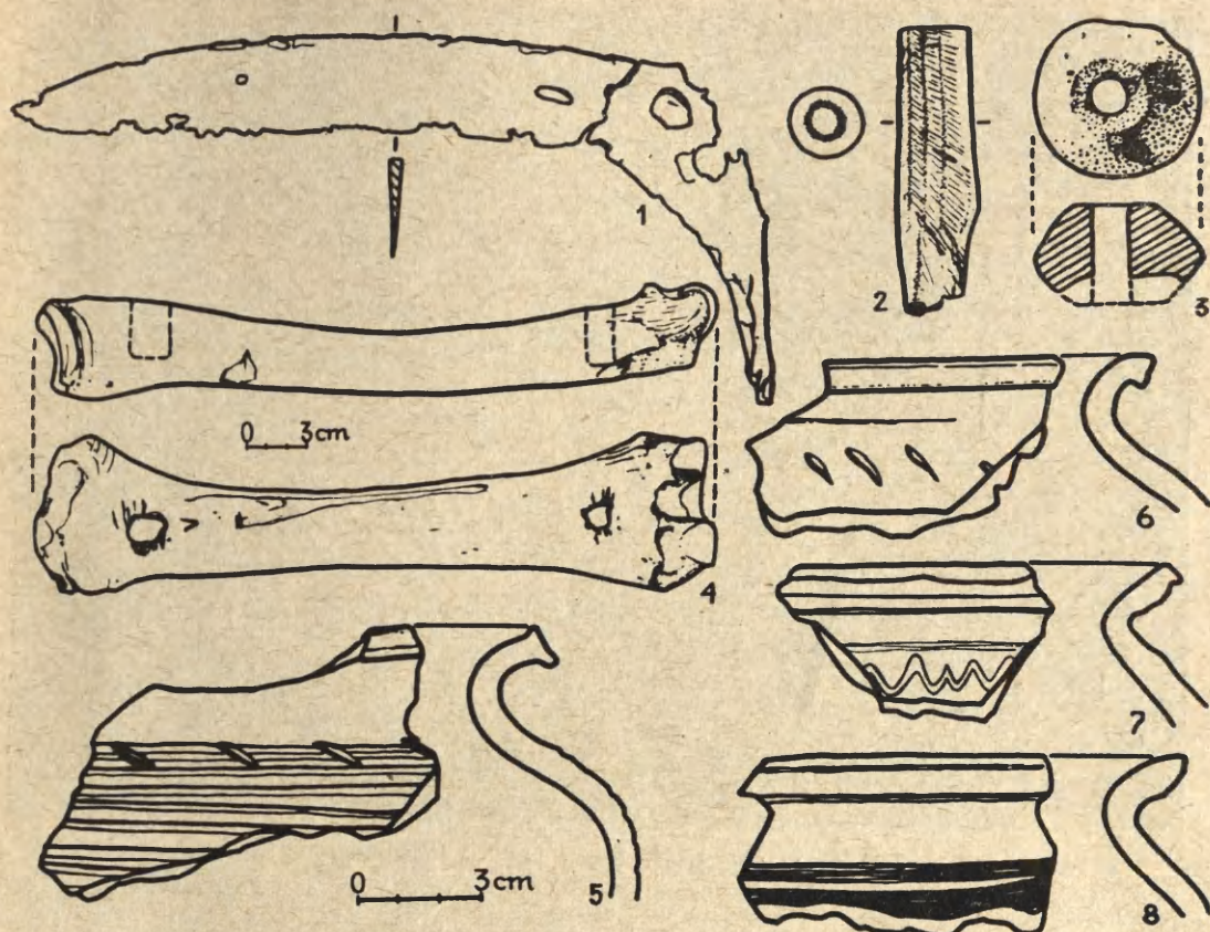
Ryc. 2. Sadowel, pow. Góra. Zabytki z grodziska
