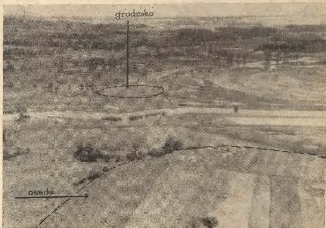
Ryc. 1. Sądowel, pow. Góra — sytuacja grodziska. Zaznaczona u dołu osada to stanowisko Czeladź Wielka
