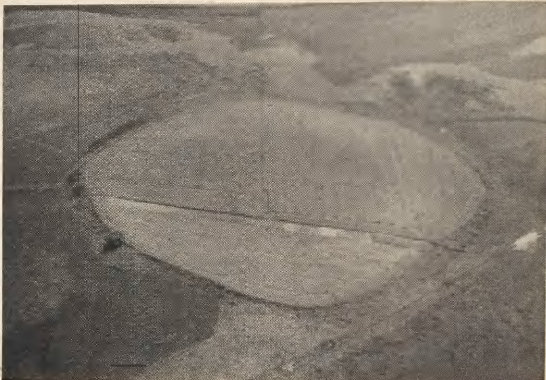
Ryc. 3. Sądowel, pow. Góra. Grodzisko
