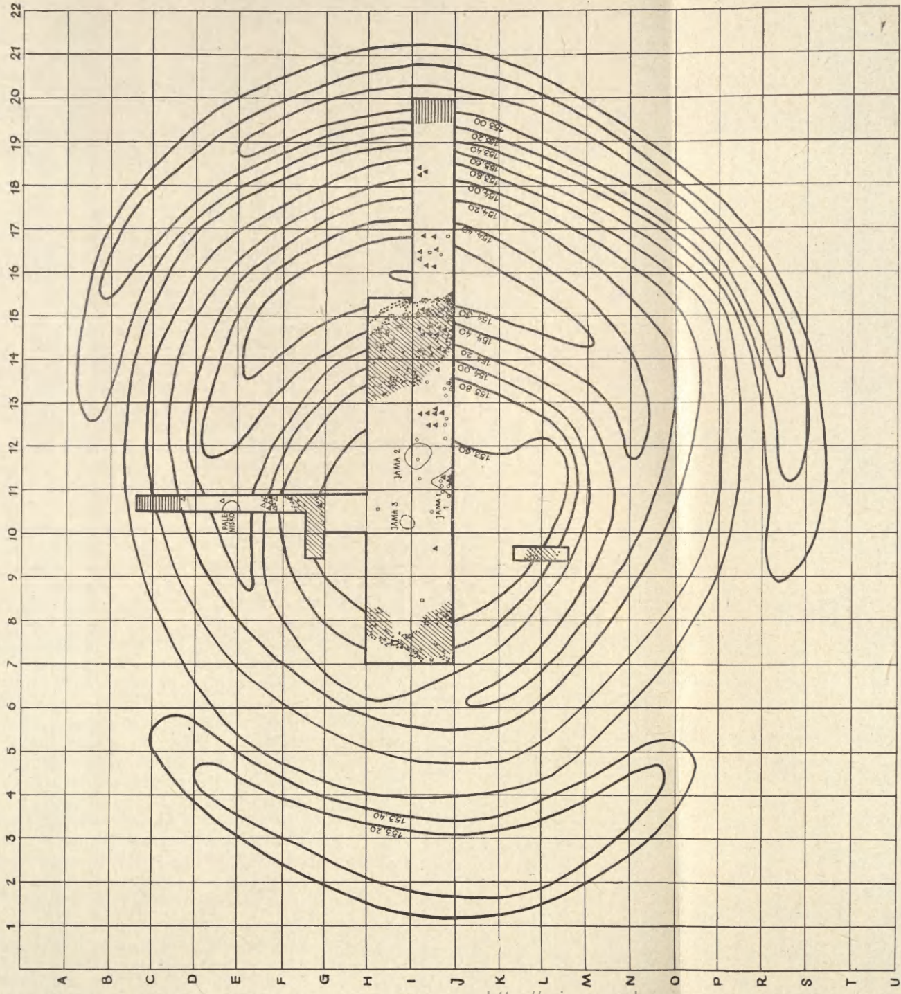
Ryc. 2. Strachów, woj. Wrocław, stan. 1. Plan stanowiska:
