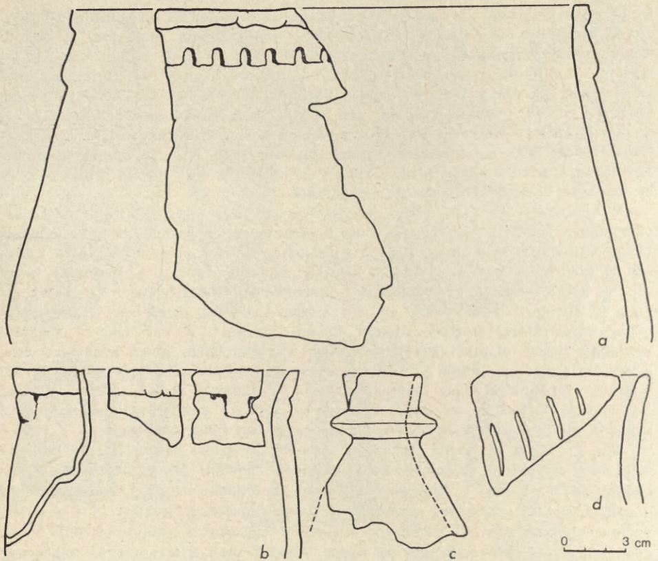
Ryc. 4. Strachów, woj. Wrocław, stan. 1. Ceramika z jamy nr 3 Pottery from pit 3
