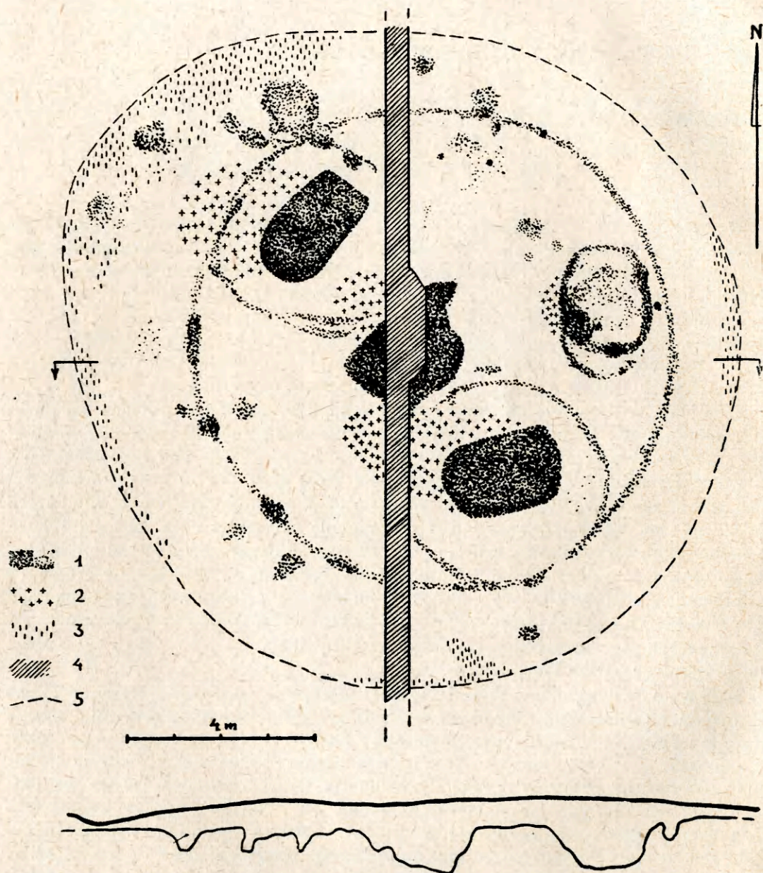
Ryc. 1. Brzezinki, pow. Lubaczów, kurhan 3. Rzut poziomy po zdjęciu nasypu kurhanowego
