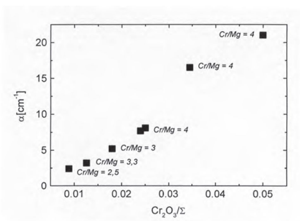
Rys. 5. Współczynnik absorpcji warstw Cr,Mg: YAG dla \lambda = 1064 nm w funkcji ułamka molowego \text{Cr}_2\text{O}_3 w roztworze. Stosunek stężeń wyjściowych \text{Cr}_2\text{O}_3 i MgO oznaczono jako Cr/Mg. Fig. 5. Absorption coefficient of Cr,Mg: YAG layers for \lambda = 1064 nm as a function of \text{Cr}_2\text{O}_3 mol fractions in the melt, where Cr/Mg denotes the mole concentration ratio of \text{Cr}_2\text{O}_3 to MgO.
