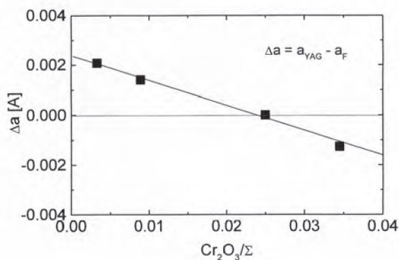
Rys. 2. Różnica stałych sieci warstwy Cr,Mg:YAG i podłoża YAG w funkcji ułamka molo-wego \text{Cr}_2\text{O}_3 w składzie wyjściowym. \text{Cr}_2\text{O}_3/\Sigma oznacza ułamek molowy \text{Cr}_2\text{O}_3 w roztworze. Fig.2. The difference between Cr,Mg:YAG film and YAG substrate lattice constant as a func-tion of \text{Cr}_2\text{O}_3 mol fractions in the melt. \text{Cr}_2\text{O}_3/\Sigma denotes \text{Cr}_2\text{O}_3 mole fraction in the melt.
