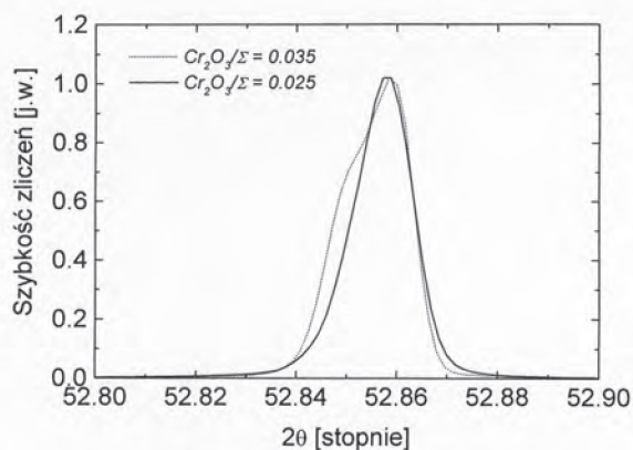
Rys. 3. Dyfraktogram struktur epitaksjalnych Cr,Mg:YAG/YAG otrzymanych przy różnej zawartości \text{Cr}_2\text{O}_3 w roztworze. Fig. 3. X-ray diffraction patterns of Cr,Mg:YAG/YAG epitaxial structures for various \text{Cr}_2\text{O}_3 mole fractions in the solution.
