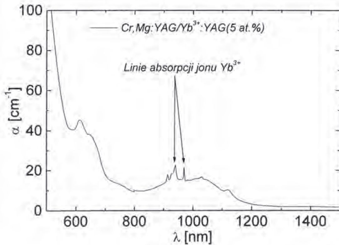
Rys. 8. Widmo absorpcyjne epitaksjalnej struktury mikrolaserowej \text{Cr,Mg:YAG/Yb:YAG} . Fig. 8. Absorption spectrum of \text{Cr,Mg:YAG/Yb:YAG} microlaser epitaxial structure.
