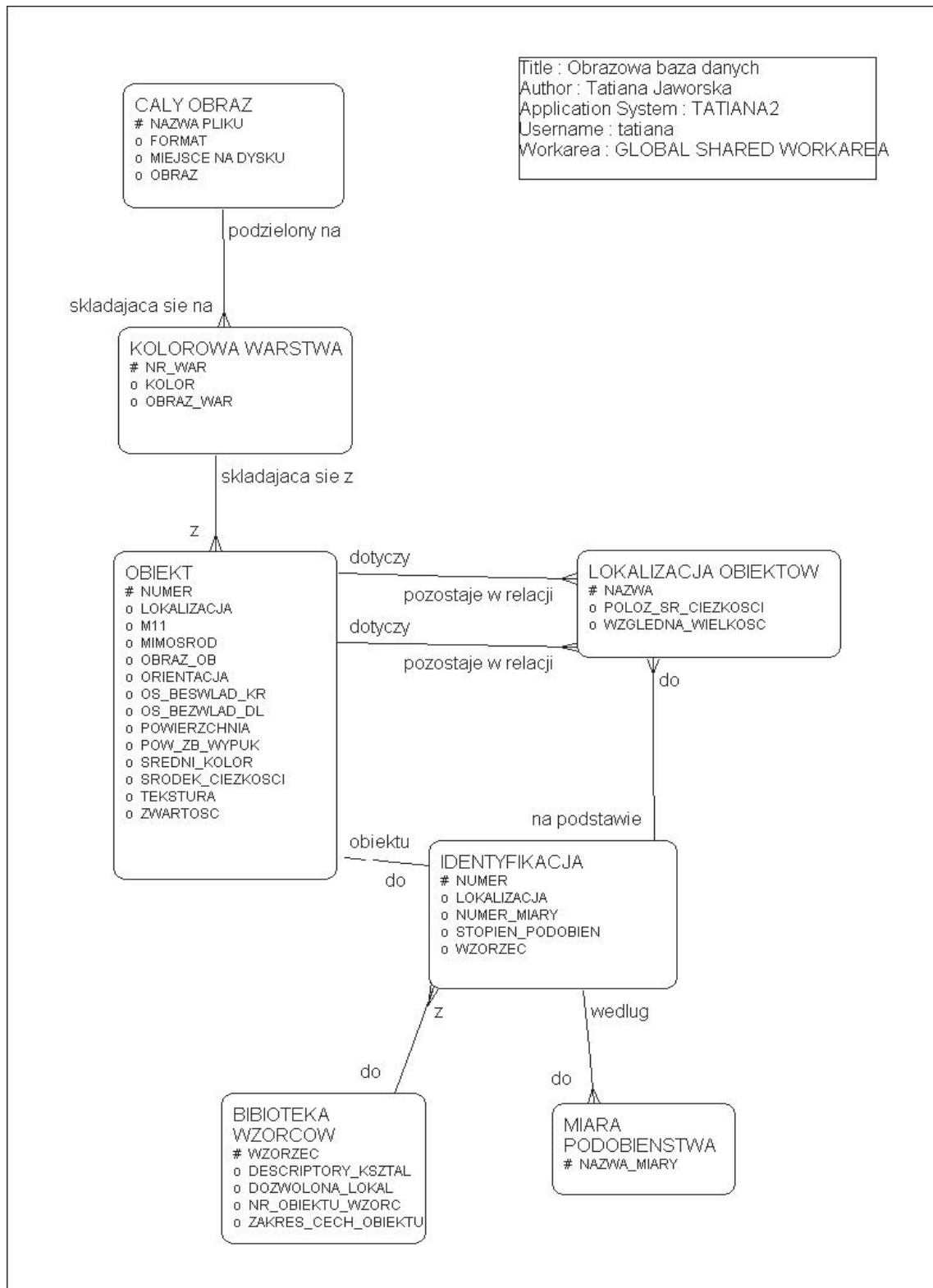
Rys. 2. Obrazowa baza danych - schemat związków encji (ERD - entity-relationship diagram).
