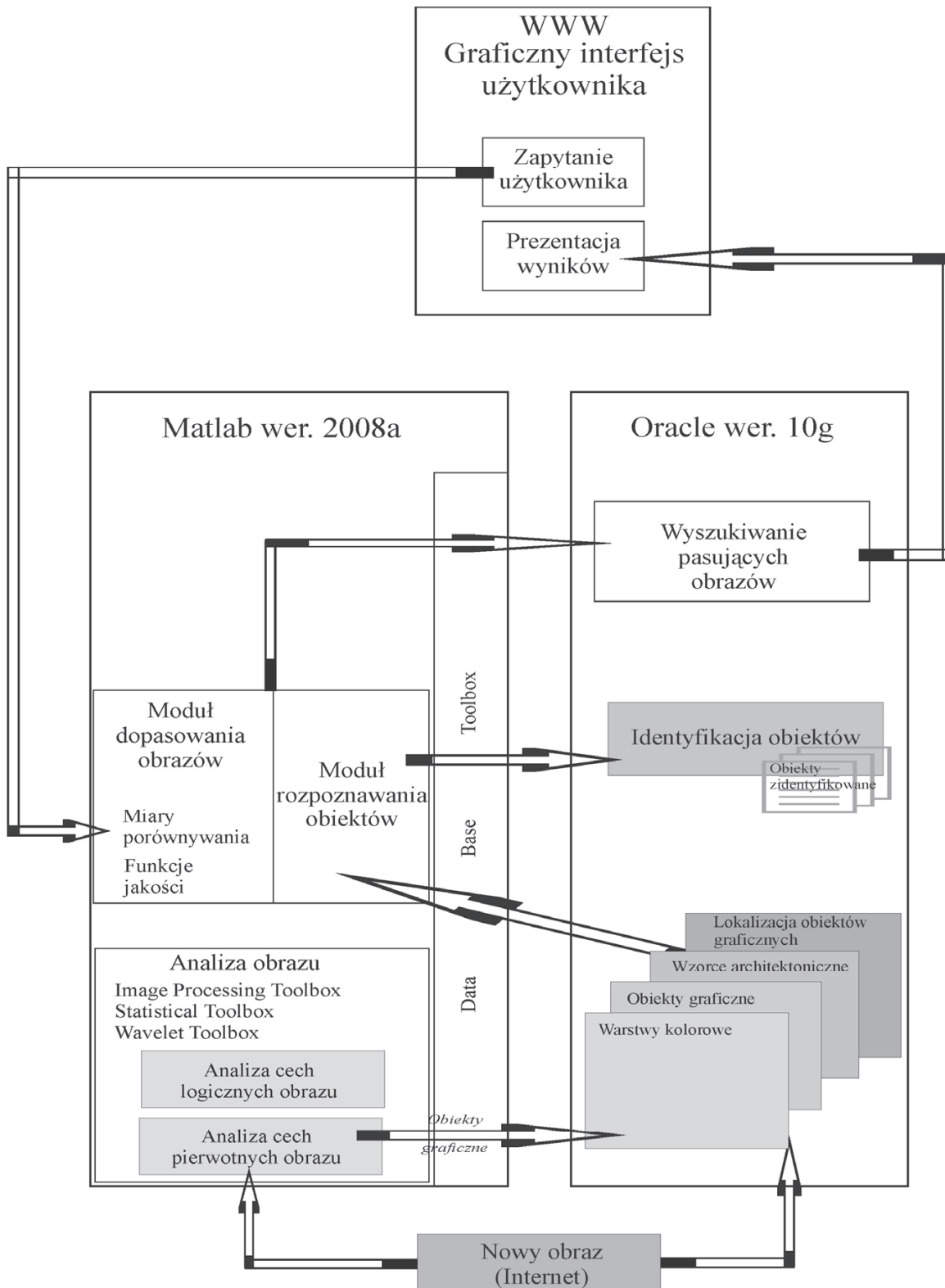
Rys. 4. Przepływ informacji pomiędzy programami Matlab i Oracle wewnątrz systemu obrazowej bazy danych.
