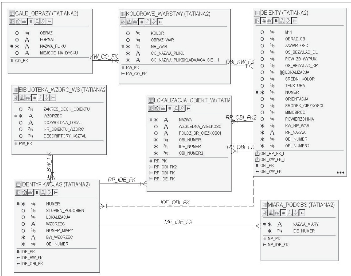
Rys. 3. Model dla serwera bazy danych Oracle 10g
