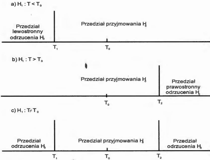
Rys. 13. Istota hipotez alternatywnych H_1 względem hipotezy zerowej H_{j0}: T = T_0 : a) hipoteza (test) lewostronna, b) hipoteza (test) prawostronna, c) hipoteza (test) obustronna.
